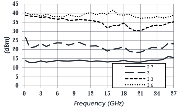
Input IP3 vs VDD - RF1/RF4
