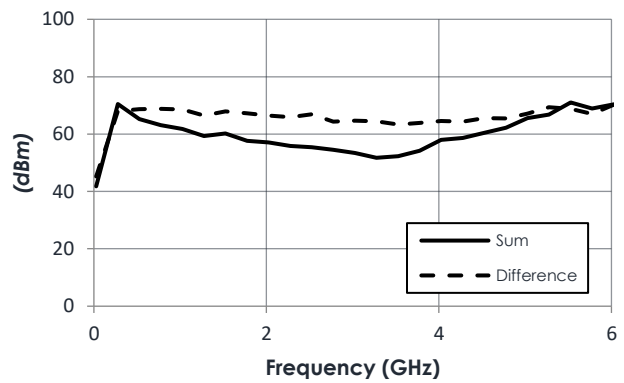
Output IP2
